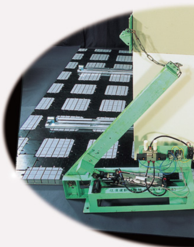
前置波・正弦波・後置波による振動試験（耐震性能）
