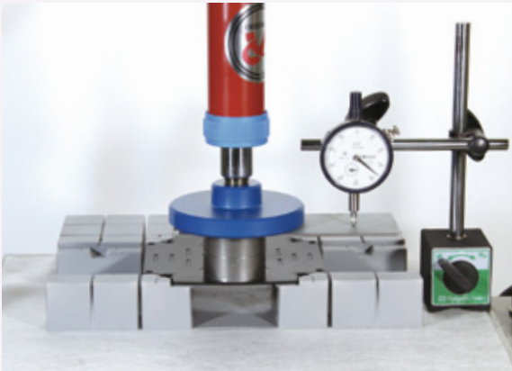
クリープ試験(許容積載荷重)
