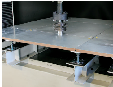
耐荷重性能試験(JIS A 1450)
