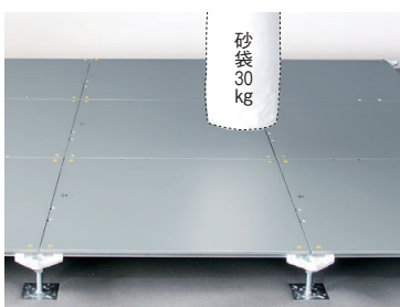
耐衝撃性能試験(JIS A 1450)
