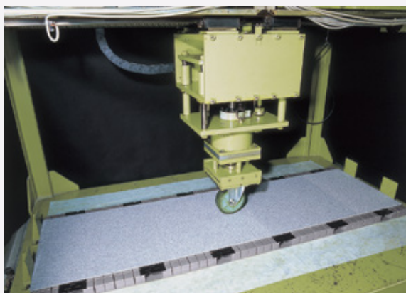
ローリングロード試験
