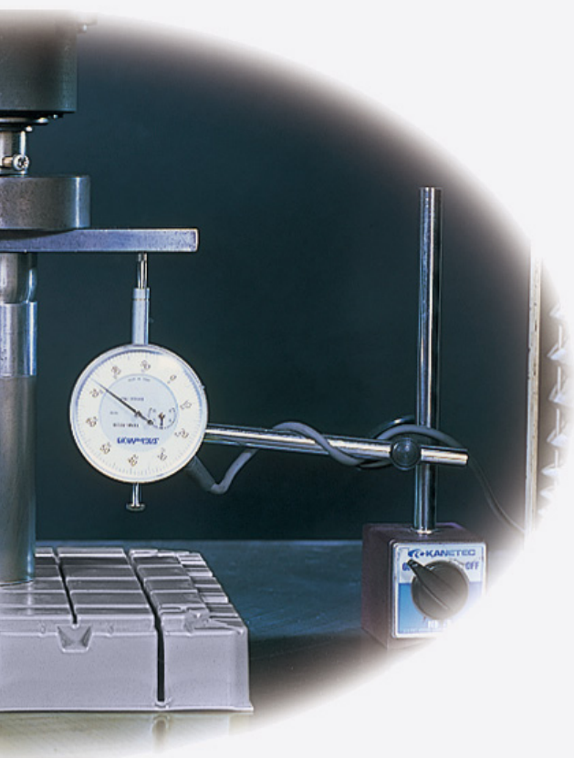
耐等分布荷重試験
