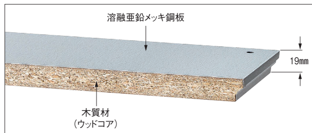
「クワッドフィックス600」 パネル断面
