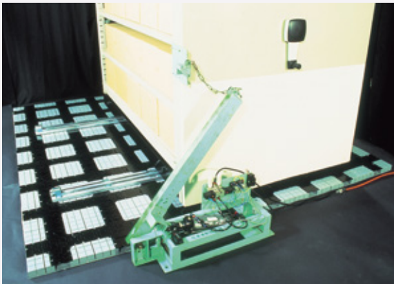
耐振動衝撃荷重試験（移動書庫）
