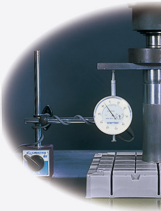
静荷重試験 (耐荷重性能)
