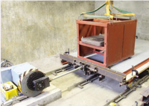
前置波・正弦波・後置波による振動試験（耐震性能）
