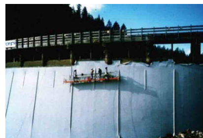
写真-2 ジオメンブレンによる漏水対策（米国） 9)
