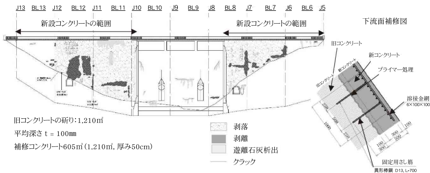
図-1 凍害によるコンクリートダム堤体表面の打替え 12)
