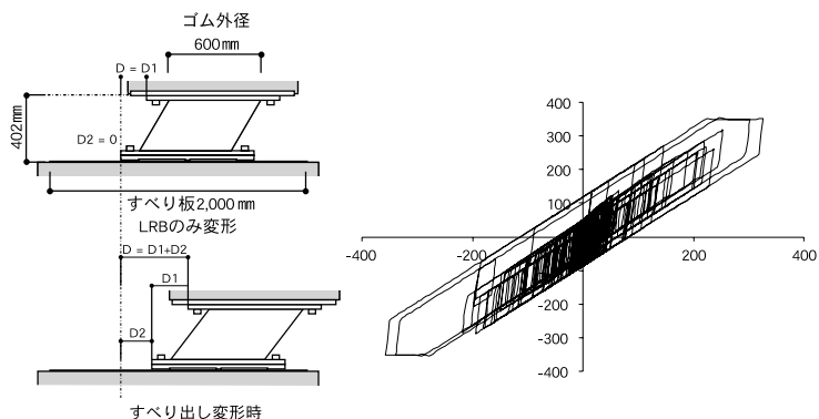
図-24 QTBの変位-水平力関係
