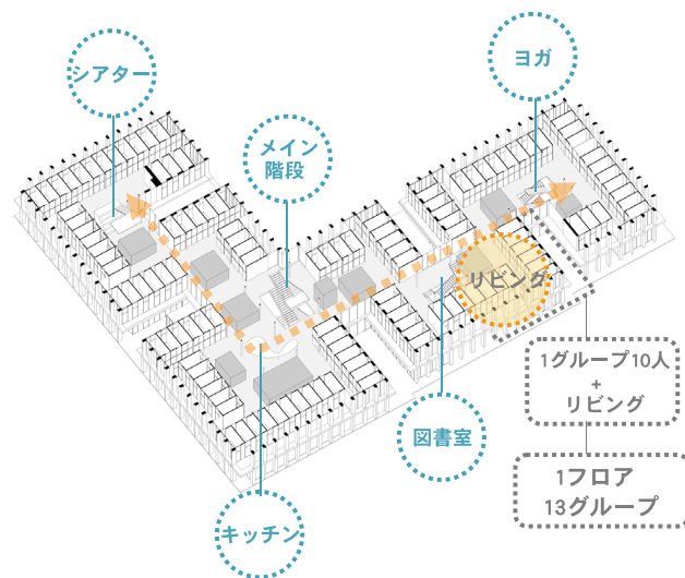
図-6 基準階アクソメ
