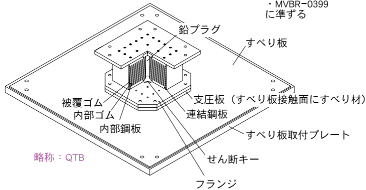
図-25 QTBの構成
