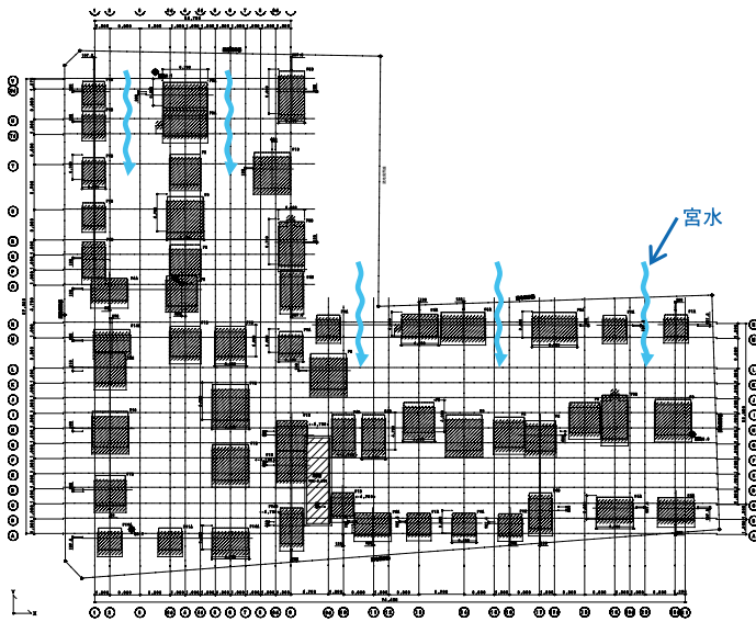
図－15 地盤改良伏図
