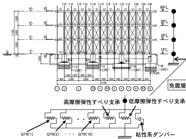
図－16 地震応答解析モデル概念図
