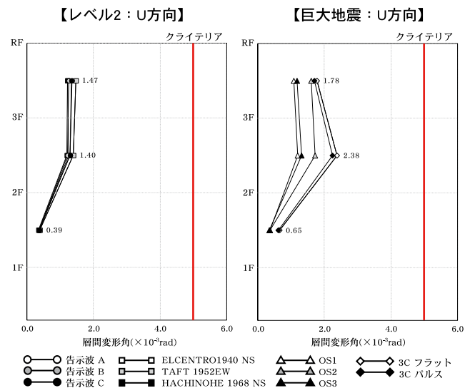
図-20 最大層間変形角
