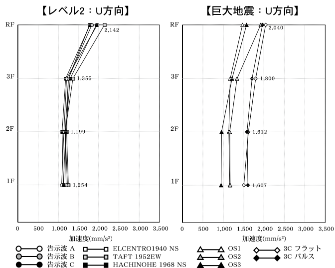
図-21 最大加速度
