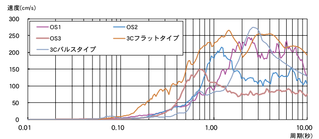
図－18 THE免震の効果検証用長周期地震動 擬似速度応答スペクトル
