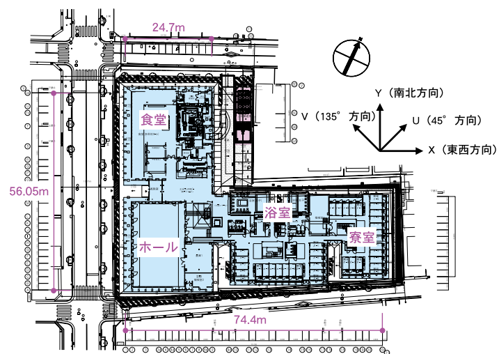
図-4 1階平面図兼配置図
