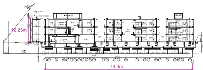
図-5 断面図
