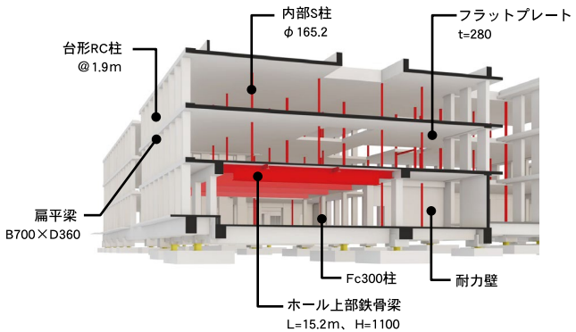
図ー８ 構造計画概要図
