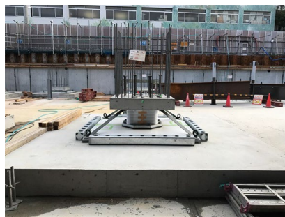
写真-5 免震材料施工写真2
