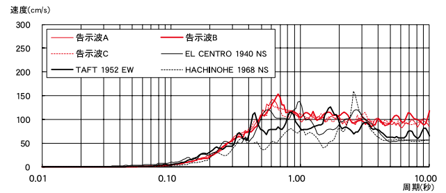
図－17 レベル2地震動 擬似速度応答スペクトル
