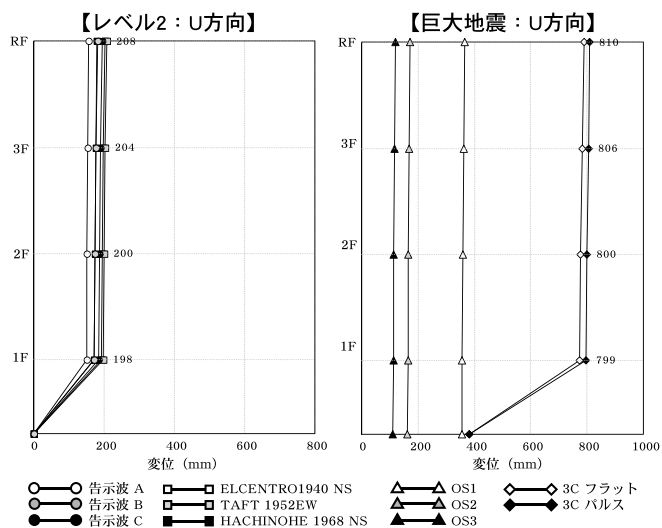
図-19 最大変位
