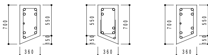
図-12 台形柱の断面
