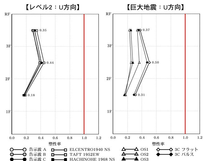
図-22 最大層間塑性率
