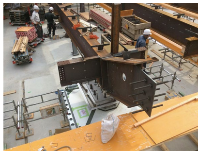
写真-6 1階SRC梁施工写真
